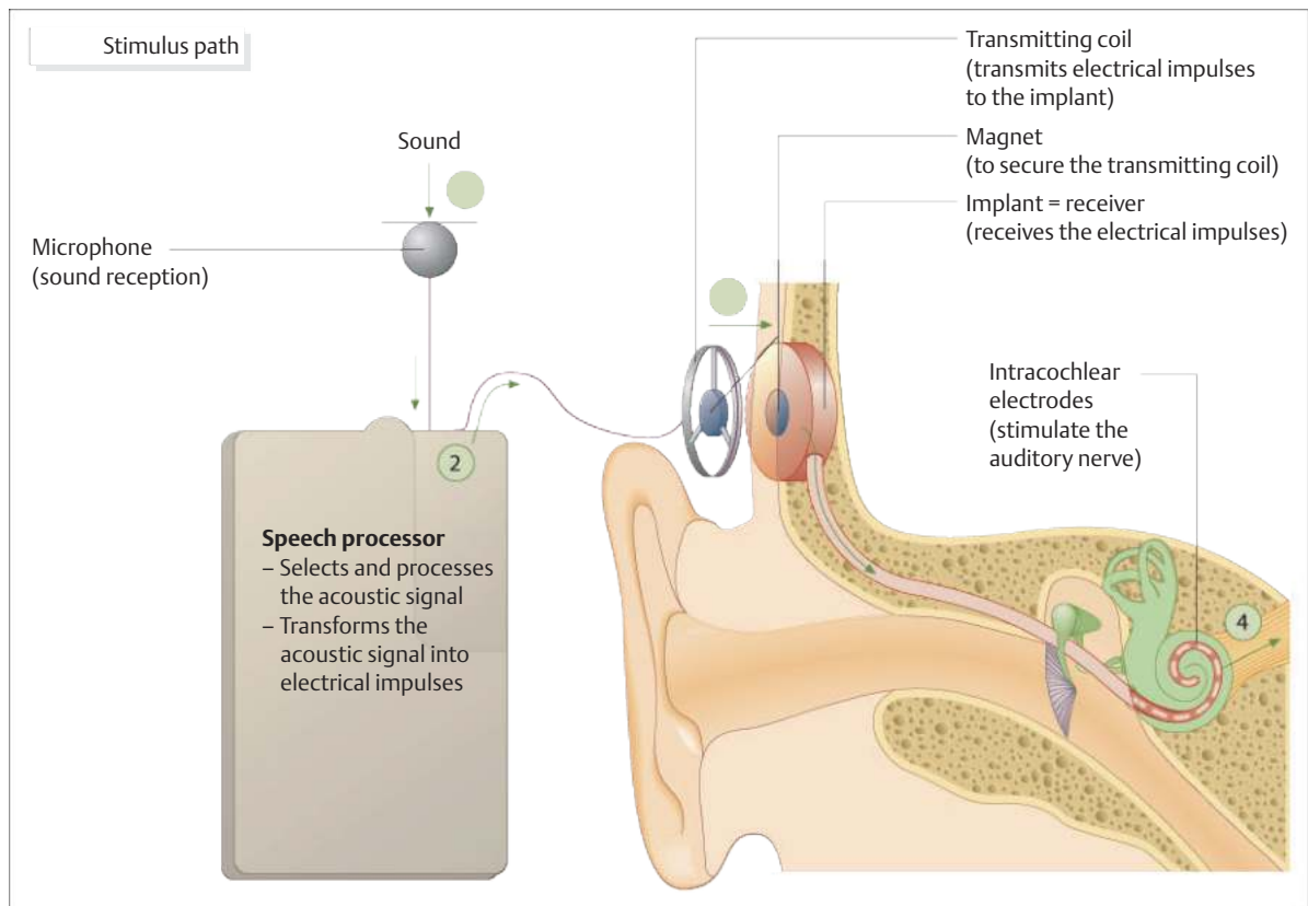
Fig. Cochlear implant (CI)
